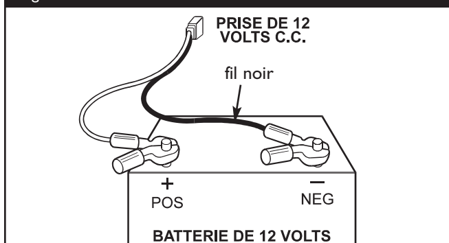
Figure 24 - Branchement des Câbles de Batterie
